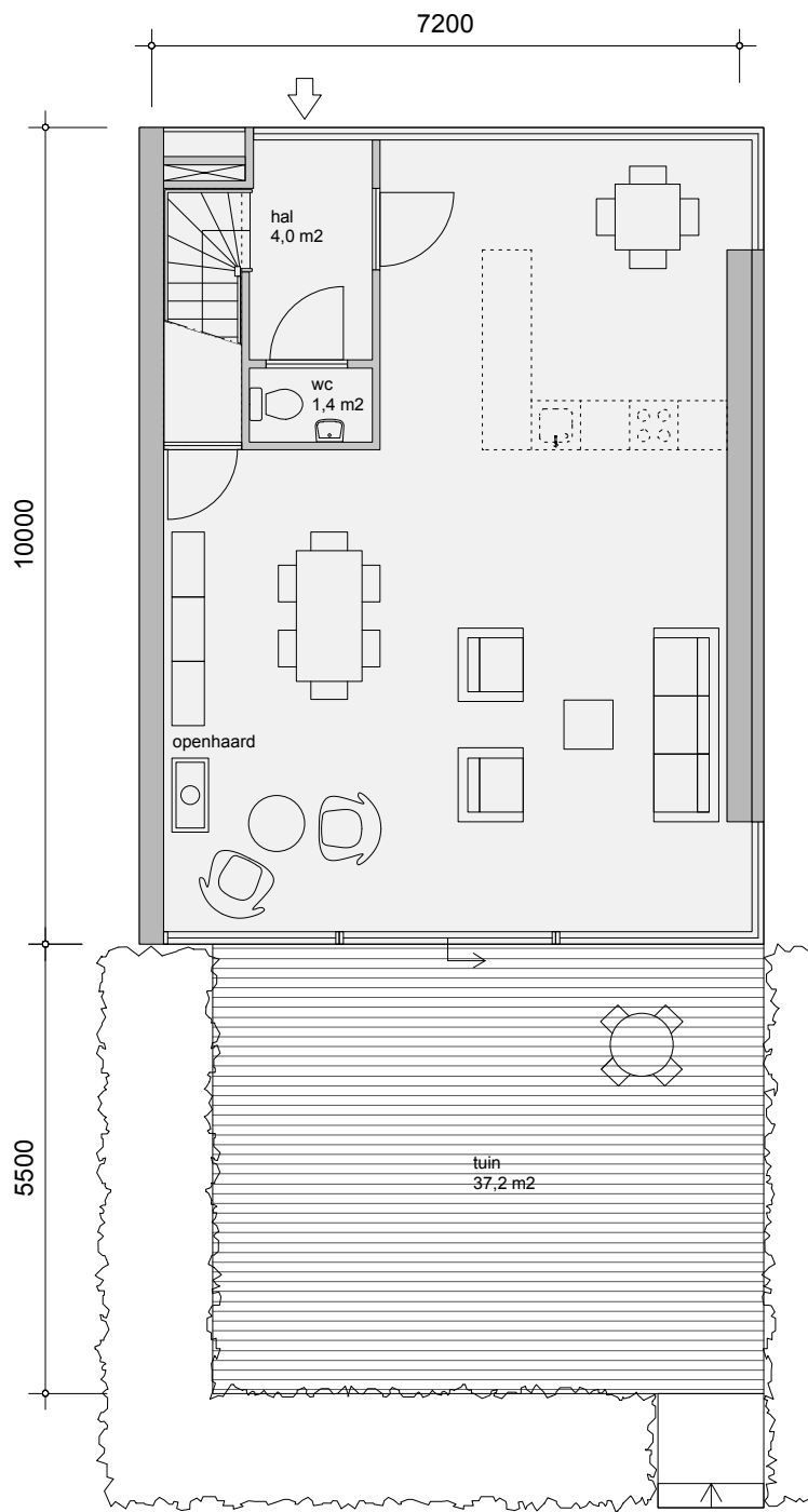
BEGANE GROND
