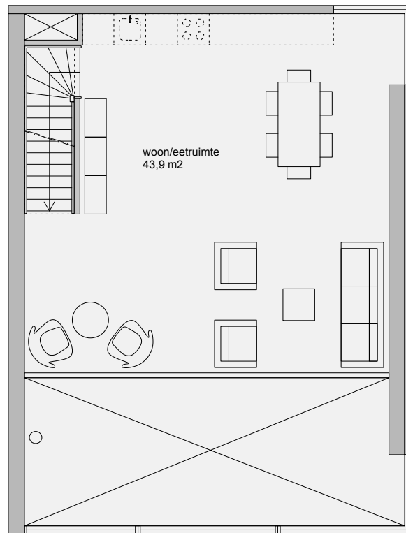
EERSTE VERDIEPING
